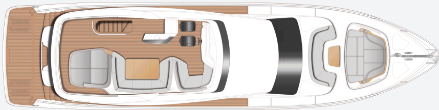
Y72 Flybridge
